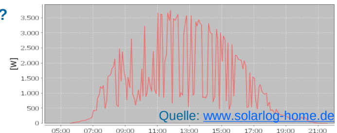
Einspeiseprofil Photovoltaik
